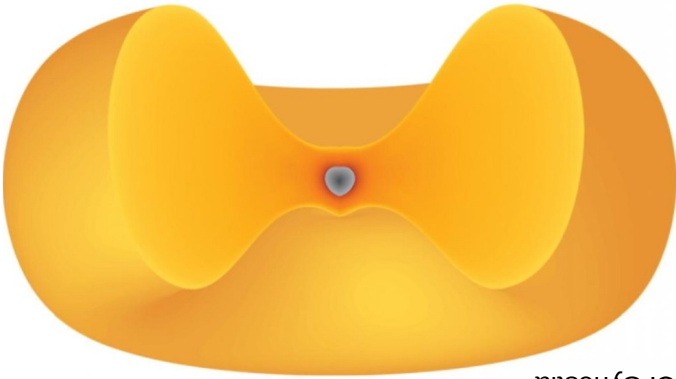
C. Synestia
