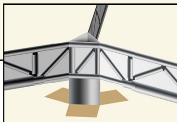
Détail sur la partie centrale des supports d'atterrissage
