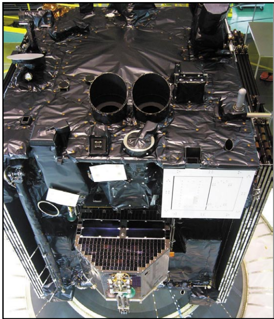
Philae fixé sur Rosetta © ESA.
