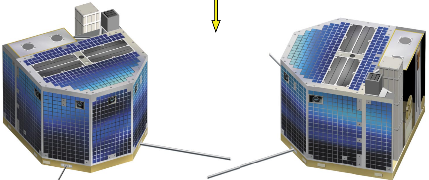
Vues de la plateforme de Philae assemblée avec ses instruments
